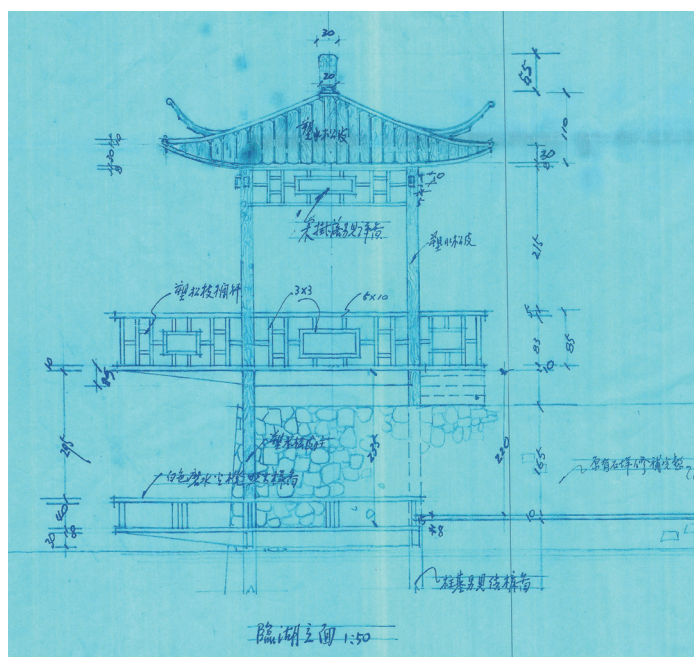
图 3 春光亭立面图（1972 年图纸）
