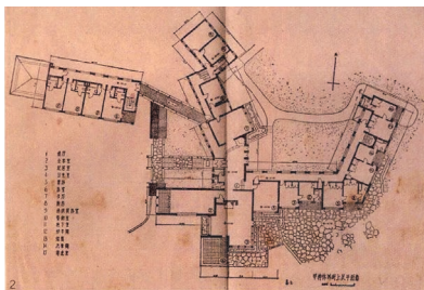
图4 武昌东湖客舍甲所和乙所的平面图
