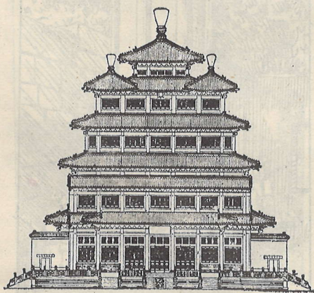
图2热河避暑山庄乘之阁南立面图
